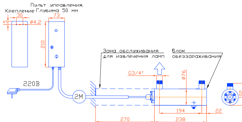
Монтажный чертёж установки КРИСТАЛЛ-0.5 Патрубки – П. Изготовление под заказ. Горизонтальное расположение
