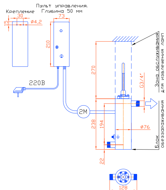
Монтажный чертёж установки КРИСТАЛЛ-0.5 Патрубки – И. Изготовление под заказ. Вертикальное расположение
