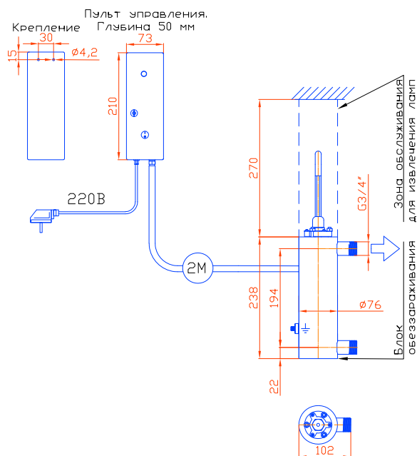
Монтажный чертёж установки КРИСТАЛЛ-0.5 Патрубки – П. Стандартное изготовление. Вертикальное расположение
