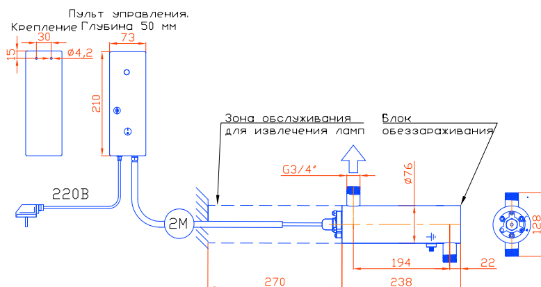
Монтажный чертёж установки КРИСТАЛЛ-0.5 Патрубки – И. Изготовление под заказ. Горизонтальное расположение
